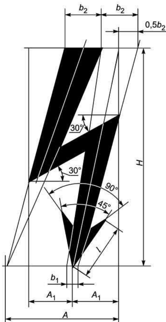
Рисунок Н.1 — Графический символ электрического напряжения
